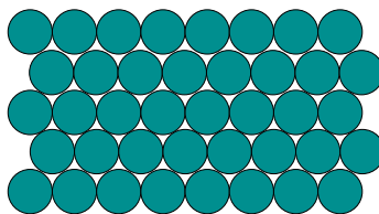
Figure 3 : empilement de disques dans le plan (densité \frac{\pi}{2\sqrt{3}} \simeq 0,9069 ).
